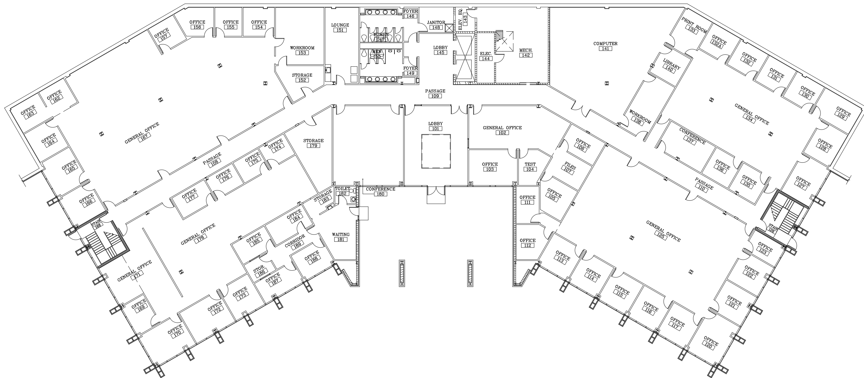
FIRST FLOOR PLAN SCALE: N.T.S.
